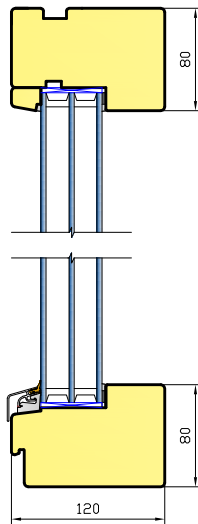
Lõige A-A 1:1
