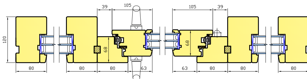
Lõige C-C 1:1
